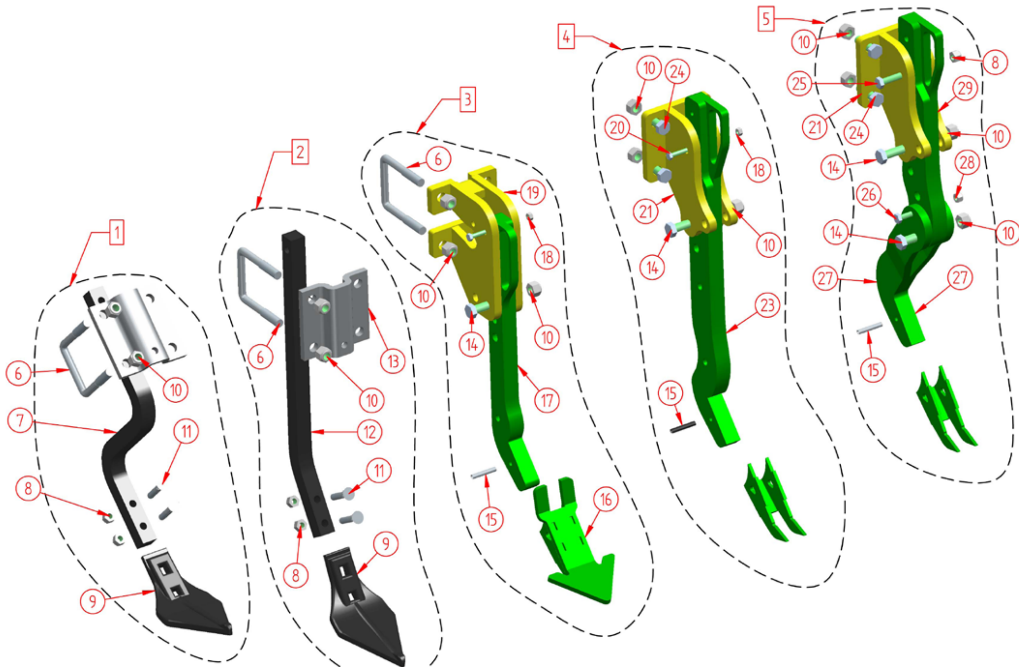
ROMPITRACCIA ERPICI - WHEEL MARK ERADICATOR
